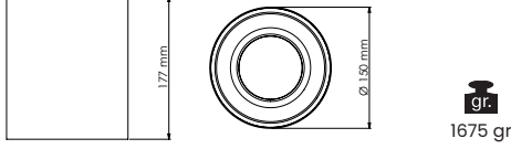
Teknik Çizim | Technical Drawing
